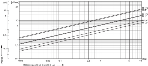
Диаграмма коэффициента k_{VS}
