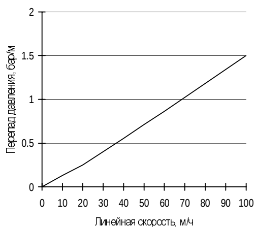
Рис. 2. Перепад давления
